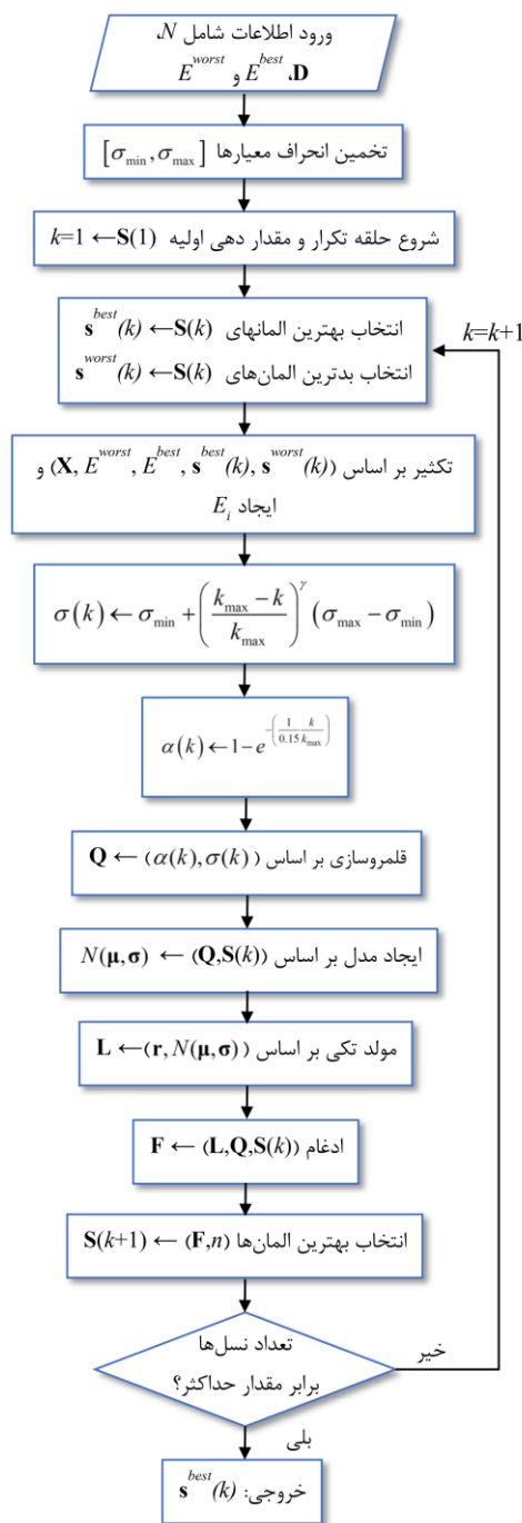
شکل (۳): فلوجارت روش بهینه‌سازی ترکیبی IWO-EDA
