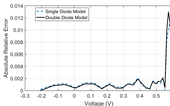
شکل (۸): مقایسه دقت دو مدل تک دیودی و دو دیودی
