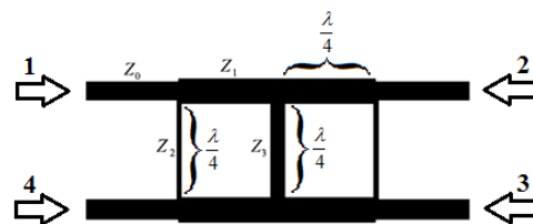
شکل (۲): تزویج کننده جهت‌دار شاخه‌ای دو بخشی پهن باند شده
