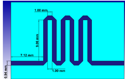
شکل (۹): تغییردهنده فاز شیفرن طراحی شده 45^\circ درجه
