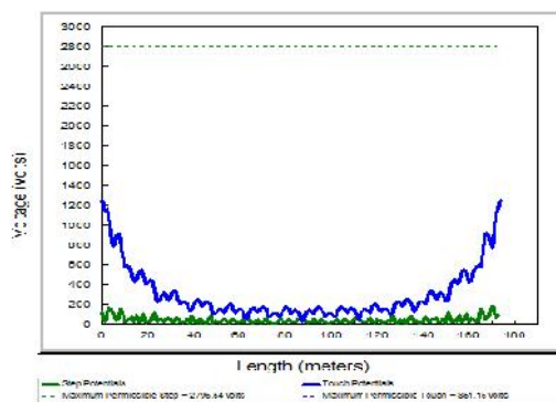
شکل (۲): پروفیل پتانسیل طرح اول سیستم زمین پست تفت
