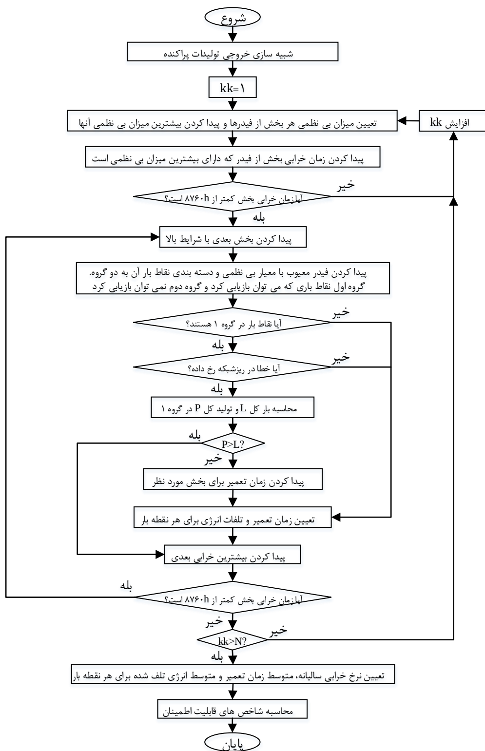
شکل (۱): فلوچارت مورد استفاده برای ارزیابی قابلیت اطمینان سیستم توزیع RBTS BUS 2 شامل تولیدات پراکنده با معیار بی نظمی
