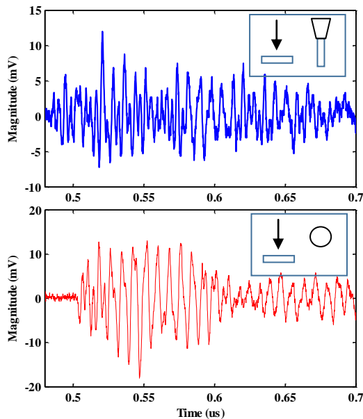
شکل (۱۲): سیگنال‌های اندازه‌گیری شده در دو حالت پلاریزاسیون مخالف (شکل بالا) و پلاریزاسیون موافق (شکل پایین)
