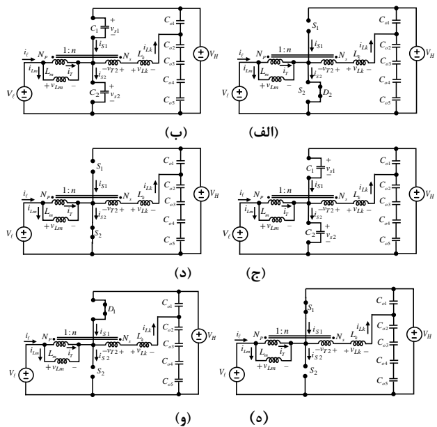
شکل (۳): مدار معادل‌های مبدل پیشنهادی برای حالت تک طبقه؛ (الف) مد کاری اول؛ (ب) مد کاری دوم (بازه زمانی t_1 \leq t < t_{D2} )؛ (ج) مد کاری دوم (بازه زمانی t_{D2} \leq t < t_{D1} )؛ (د) مد کاری سوم؛ (ه) مد کاری چهارم (بازه زمانی t_3 \leq t < t_{D1} )؛ (و) مد کاری چهارم (بازه زمانی t_{D1} \leq t < t_4 )
