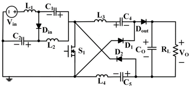
شکل (۱): مبدل شبه منبع امپدانس پیشنهادی
