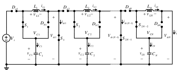
شکل (۱۰): مدار معادل ساختار پیشنهادی N طبقه و در بازه زمانی 0 \leq t \leq D_{ST}T_s
