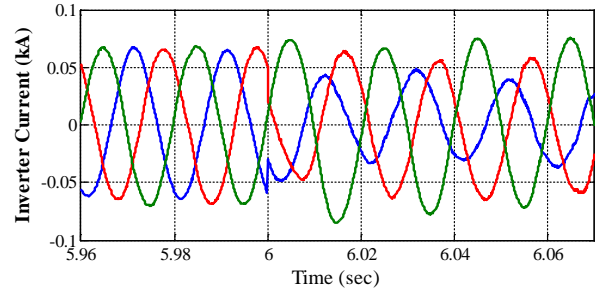
شکل (۸) شکل موج جریان سه فاز خروجی اینورتر
