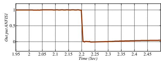
شکل (۱۵): ارزیابی امنیت ریزشبهه مورد مطالعه در هنگام اختلالات توان و بار با استفاده از ANFIS1
