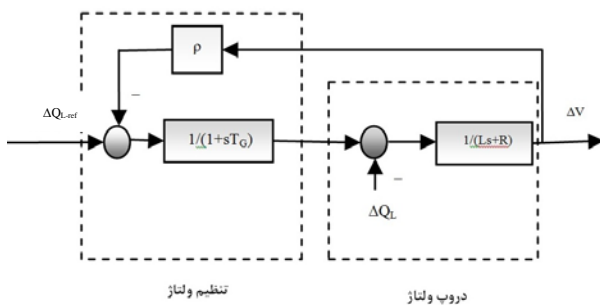
شکل (۲): نمودار بلوکی کنترلر ولتاژ- توان واکنشی برای یک واحد تولیدپراکنده با واسط الکترونیک قدرت [۲۵]
