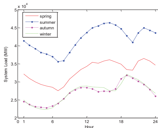
شکل (۱): تغییرات منحنی بار یک روز نمونه از هفته در فصول مختلف سال ۹۲ برای کشور ایران
