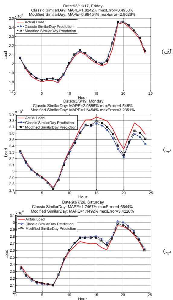
شکل (۳): تاثیر استفاده از شاخص اولویت‌بندی و بخش‌بندی سیستم قدرت برای سه روز متفاوت از هفته در سه فصل مختلف
