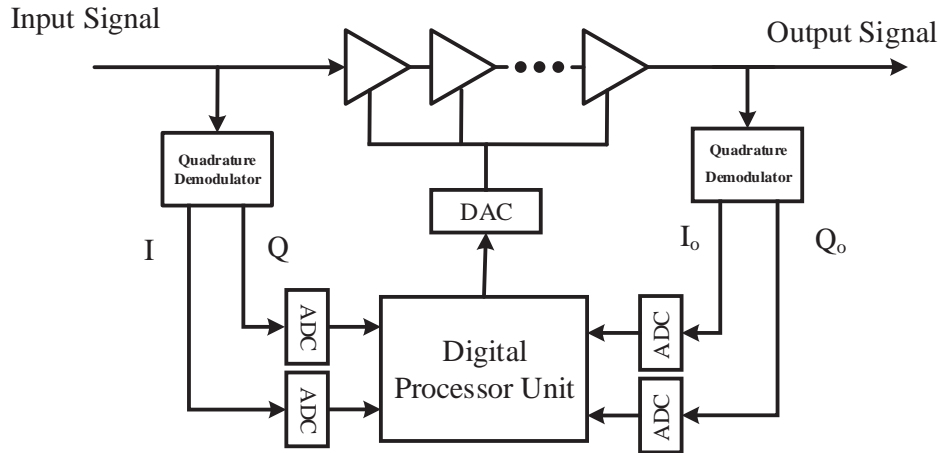
شکل (۲): ساختار دیجیتالی پیشنهادی برای حلقه‌های قفل شده تاخیر آنالوگ
