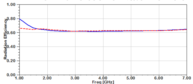
شکل (۱۵): راندمان تشعشی آنتن ارائه شده در شکل ۱
