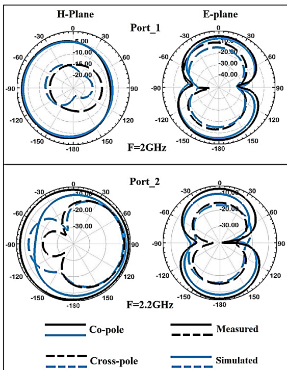
شکل (۱۲): الگوهای تشعشعی H-plane و E-plane آنتن پیشنهادی
