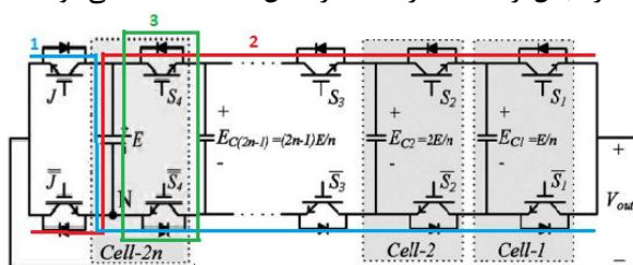
شکل (۱۴)، ساختار کلی DFCM ارائه داده شده در (۲۲)
