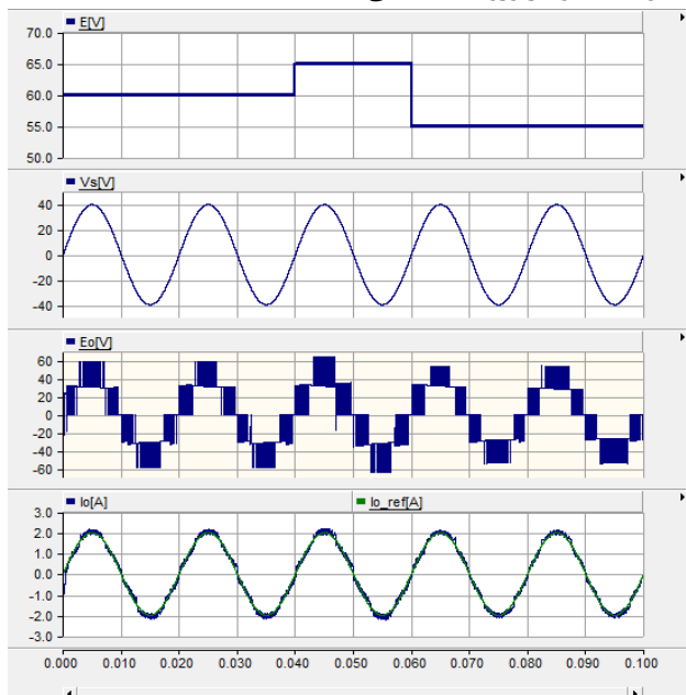
شکل (۱۶): به ترتیب از بالا به پایین، ولتاژ ورودی ( E )، ولتاژ شبکه ( V_s )، ولتاژ خروجی مبدل ( E_o ) و جریان خروجی مبدل ( I_o )
