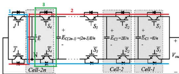
شکل (14)، ساختار کلی DFCM ارائه داده شده در (22)
