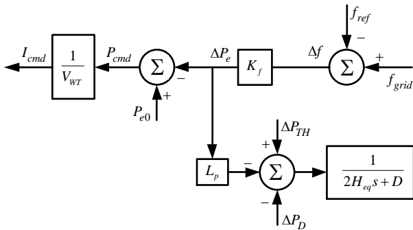
شکل (۴): حلقه کنترل تکمیلی توربین باد
