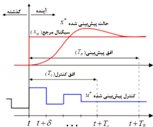
شکل (۳): قاعده کلی مدل کنترل پیش‌بین
