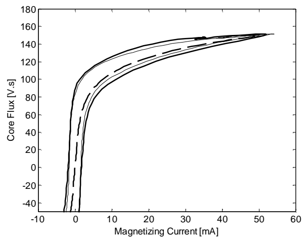
شکل ۷- مشخصه مغناطیسی مدل پیشنهادی در مقایسه با هیستریزیس اندازه گیری شده
