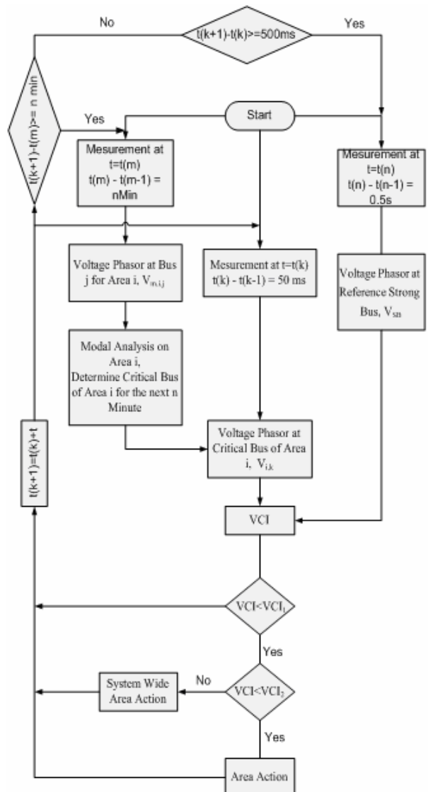
شکل ۱۳- فلوجارت الگوریتم VCI
