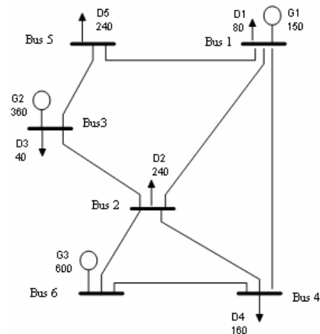
شکل (2): شماتیک سیستم تست گارور اصلاح شده
