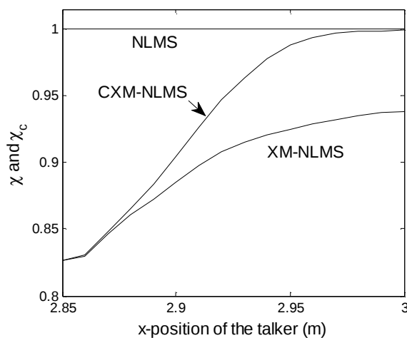
شکل (8): مقایسه مقدار c و c_e برای الگوریتمهای NLMS، CXM-NLMS و XM-NLMS
