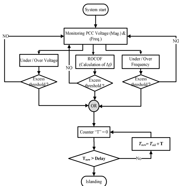
شکل (۲): فلوجارت تشخیص جزیره‌ای با استفاده از روش ترکیب رله های OFP / UFP، OVP / UVP و ROCOF
