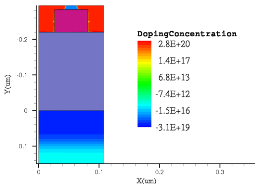
شکل (۱۱): شکل نهایی نواحی سورس و درین ترانزیستور
