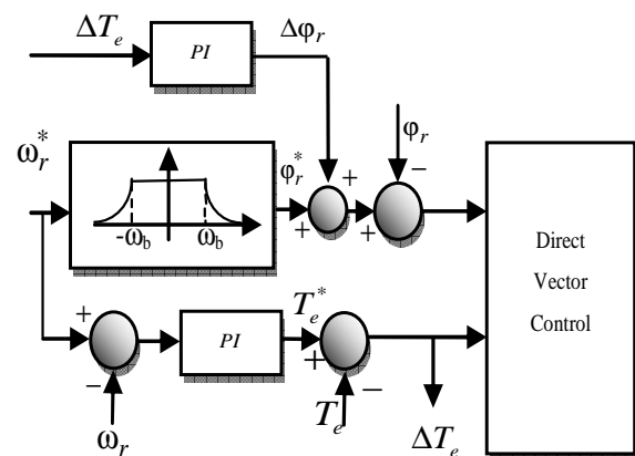
شکل (۵): بلوک دیگرام مربوط به جبران شار روتور.
