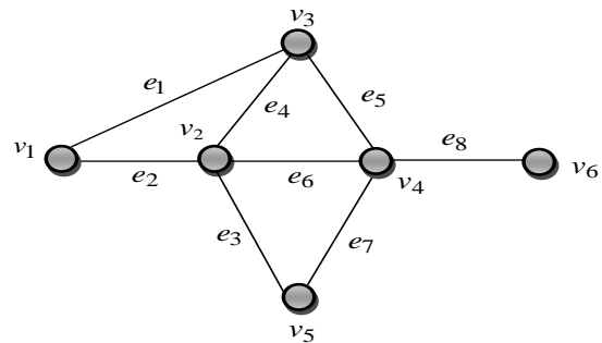
شکل (۱): نمایش اجزای یک گراف وزن‌دار ساده.
