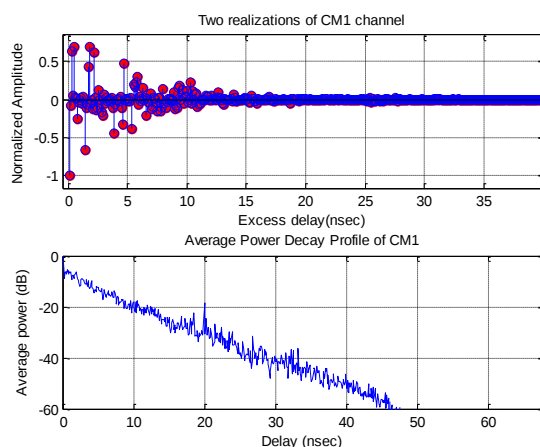
شکل (۶): کانال چند مسیر CM1 به همراه پروفایل تاخیر توان آن.
