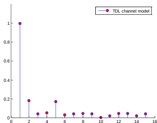
شکل (۲): کانال چند مسیر با مدل TDL شامل ۱۵ تپ
