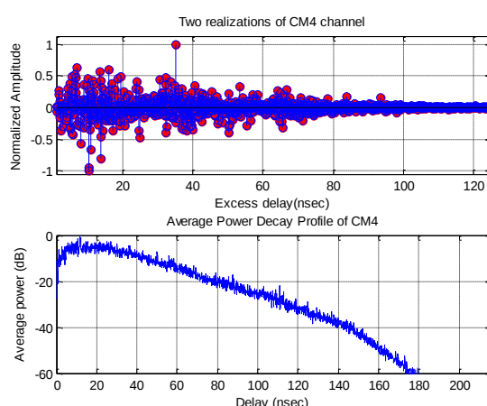
شکل (۷): کانال چند مسیر CM4 به همراه پروفایل تاخیر توان آن.
