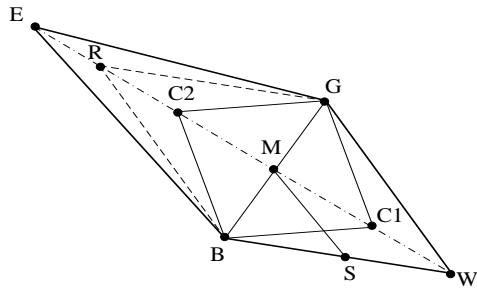
شکل (۱): الگوریتم Nelder-Mead
