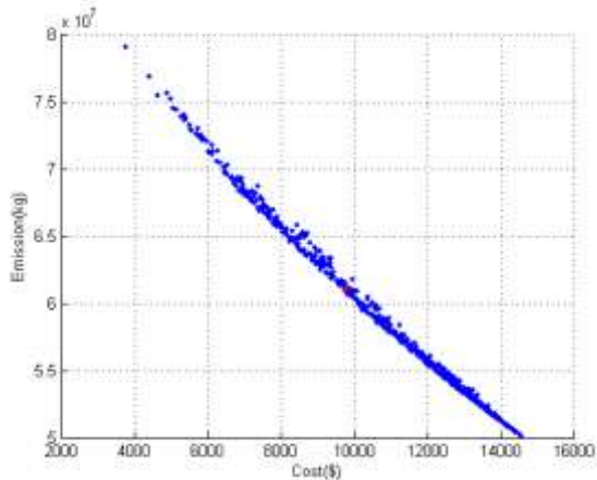
شکل (۹): منحنی پارتو هزینه-آلاینده
