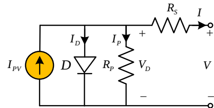
شکل (۱): مدل مدار معادل تک دیودی سلول خورشیدی
