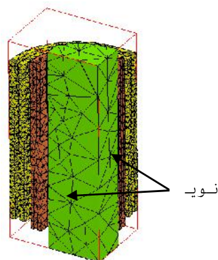
شکل (۶): شرایط مرزی مدل ترانسفورماتور آوال
