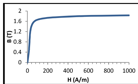
شکل (۳): منحنی مشخصه‌ی مغناطیسی ترانسفورماتور
