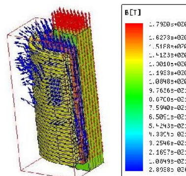
شکل (۷): بردارهای چگالی شار مغناطیسی ترانسفورماتور آوال
