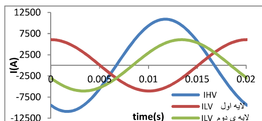
شکل (۴): منحنی جریان سیم پیچ‌های ترانسفورماتور اول و سیلندری در شرایط عملکرد نرمال
