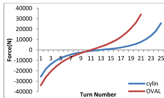
شکل (۱۶) نیروی محوری سیم پیچ HV در حالت اتصال کوتاه ترانسفورماتورهای اُوال و سیلندری
