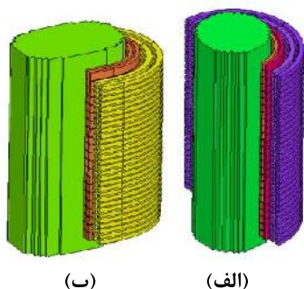
شکل (۵) مدل یک ساق ترانسفورماتور (الف) سیلندری (ب) اول
