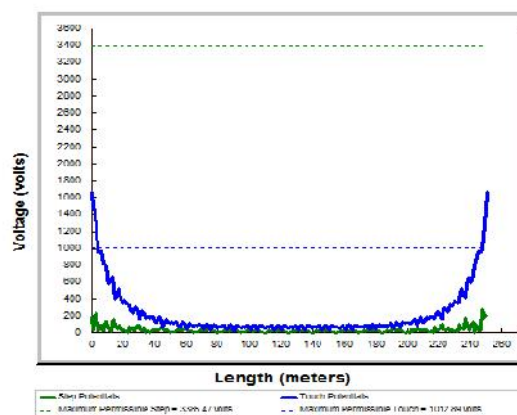
شکل (۵): پروفیل پتانسیل طرح اول سیستم زمین پست 230/63 KV
