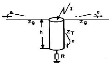
(الف): برخورد صاعقه به نوک دکل
