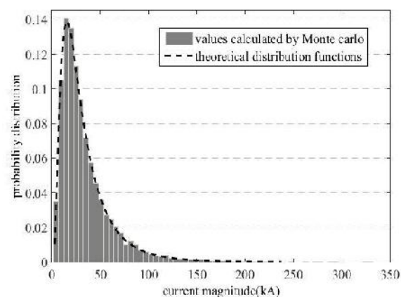
الف) توزیع مقدار دامنه جریان
