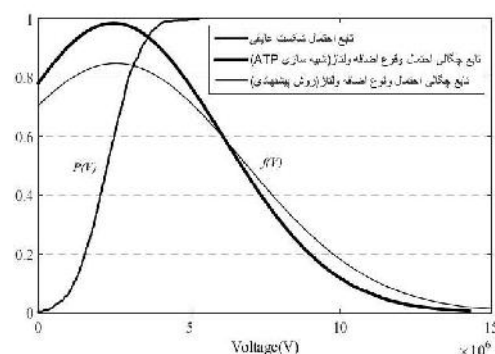
شکل (۱۲): احتمال شکست عایقی
