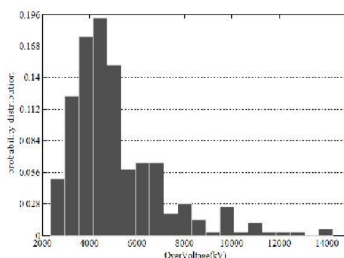
(الف) شبیه‌سازی ATP
