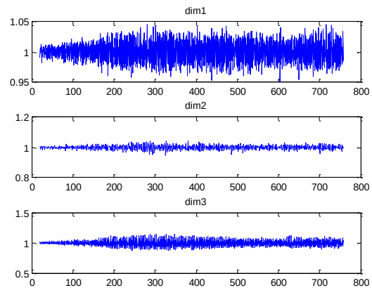
شکل (۳): محاسبه گین برای هر باند تصویر شکل (۲) به روش انطباق گشتاور با تخمین گر بهره تطبیقی با پنجره گوسین به طول ۹ ( L=4 ) (محور افقی شماره ستون تصویر و محور عمودی مقدار تخمین گین را نشان می‌دهد).
