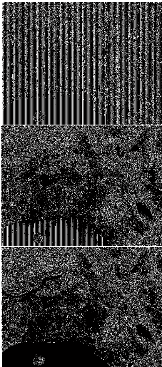
شکل (۸): (الف) لبه‌های آشکار شده در تصویر اولیه دارای خطای نوارشدگی. (ب) آشکارسازی لبه‌های آشکار شده در تصویر به روش انطباق گشتاور افقی (مبتنی بر بهره). (ج) آشکارسازی لبه در تصویر حاصل از اجرای روش پیشنهادی (مبتنی بر انحراف)
