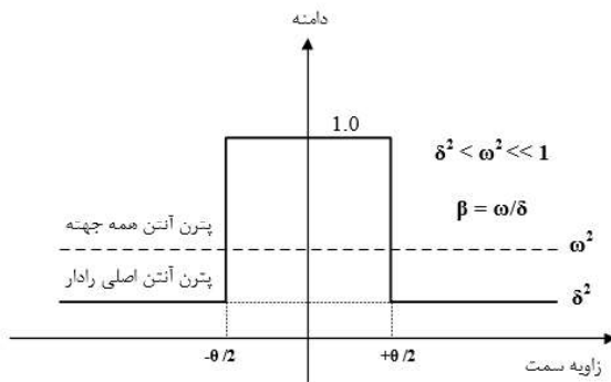
شکل (۵): پترن نرمالیزه ایده‌آل آنتن‌های اصلی و کمکی
