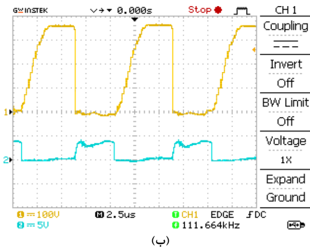
شکل (۵): شکل موج های ولتاژ(بالا) و جریان (پایین) کلید (الف) شکل موج شبیه سازی (ب) شکل موج ساخت
