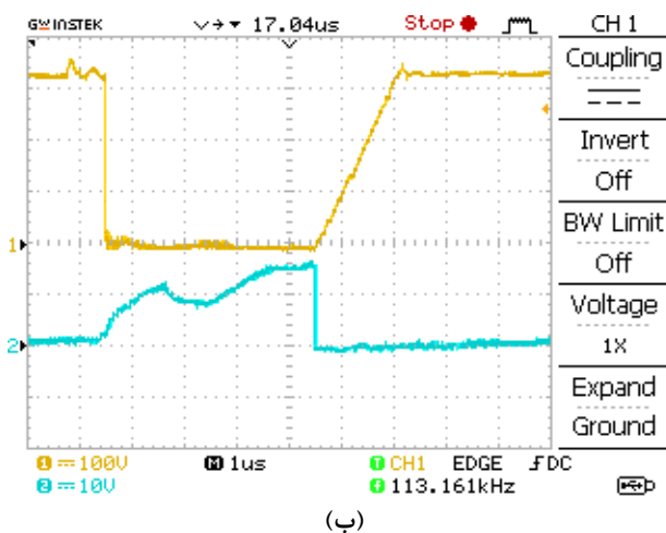
شکل (۶): شکل موج های زوم شده ولتاژ(بالا) و جریان (پایین) کلید (الف) شکل موج شبیه سازی (ب) شکل موج ساخت
