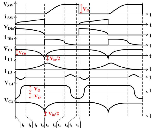
شکل (۲): شکل موج های تئوری مبدل شبه منبع امپدانس
