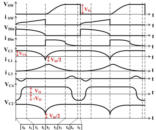
شکل (۲): شکل موج های تئوری مبدل شبه منبع امپدانسی پیشنهادی
