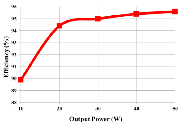
شکل (۱۱): نمودار راندمان مبدل پیشنهادی بر حسب توان های خروجی مختلف
