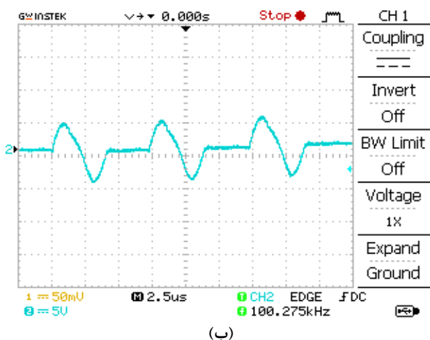
شکل (۱۰): شکل موج جریان سلف تشدید L_3 (الف) شکل موج شبیه سازی (ب) شکل موج ساخت
