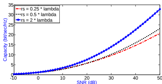
شکل (۹): ظرفیت کانال MIMO 4×4 برای فاصله ی بین آرایه ی آنتنی متغیر در سمت BS ( r_u = 0.5\lambda )
