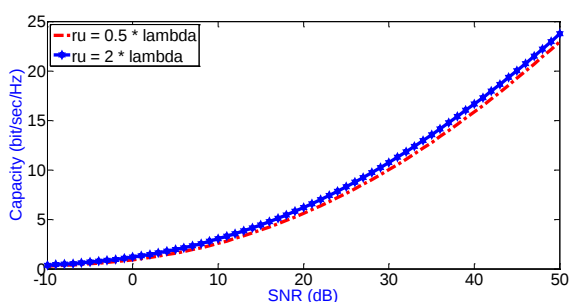
شکل (۱۱): ظرفیت کانال MIMO 4×4 برای فاصله ی بین آرایه ی آنتنی متغیر در سمت MS ( r_s = 0.5\lambda )
