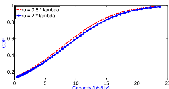
شکل (۱۲): نمودار تابع توزیع تجمعی ظرفیت کانال MIMO 4×4 برای فاصله ی بین آرایه ی آنتنی متغیر در سمت MS ( r_s = 0.5\lambda )
