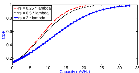
شکل (۱۰): نمودار تابع توزیع تجمعی ظرفیت کانال MIMO 4×4 برای فاصله ی بین آرایه ی آنتنی متغیر در سمت BS ( r_u = 0.5\lambda )
