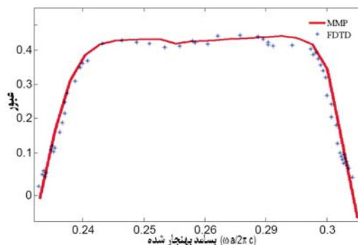
شکل (۶): میزان پرتو منتشر شده در هر شاخه جداکننده توان بهینه با دو روش FDTD و MMP
