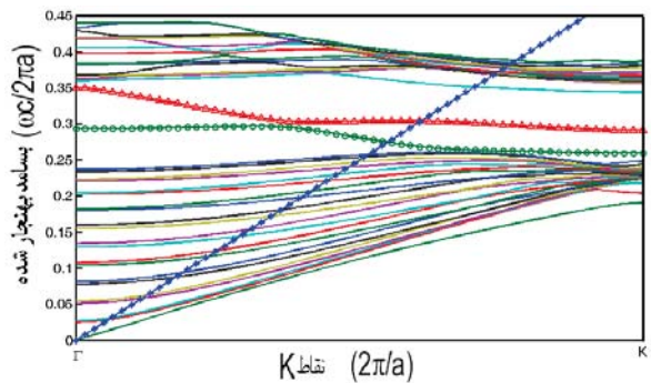
شکل (۱): ساختار نواری بلور فوتونیک، نوار ممنوعه و مدهای موجبر به وضوح قابل مشاهده هستند
