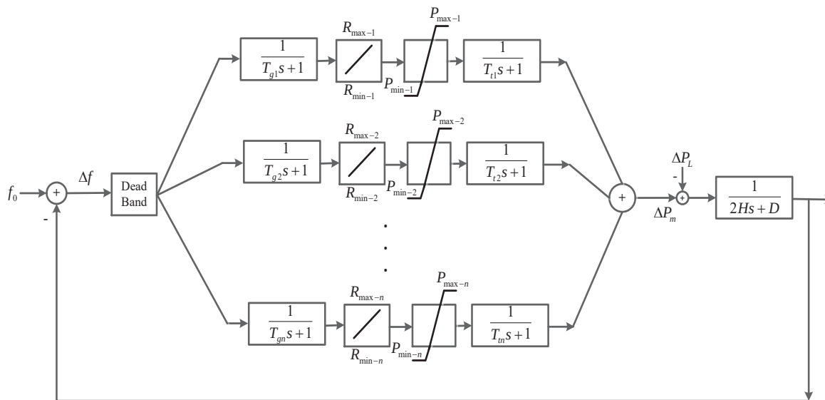
شکل (۷): مدل SFR یک سیستم قدرت با چندین واحد مشارکت کننده در کنترل فرکانس
