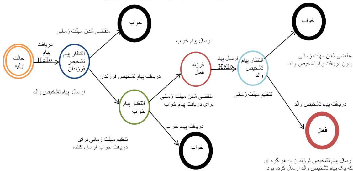
شکل (۳): ماشین حالت متناهی نشان دهنده تغییرات در الگوریتم EA-CDS
