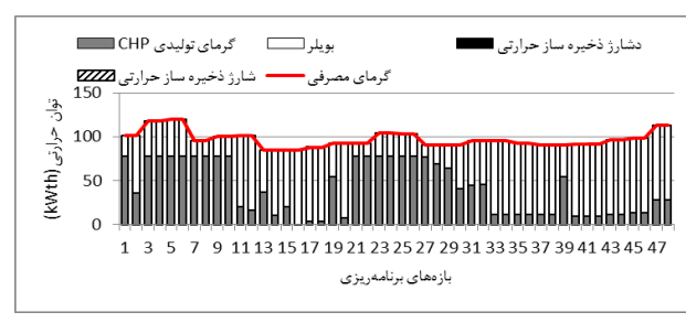
شکل (۷): سناریو ۱: تعادل توان حرارتی در ساختمان ۱
