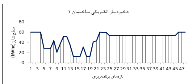
شکل (۲۱): سناریو ۳: سطح شارژ ذخیره‌ساز الکتریکی ساختمان ۱
