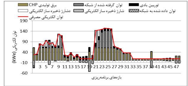
شکل (۵): سناریو ۱: تعادل توان الکتریکی در ساختمان ۱
