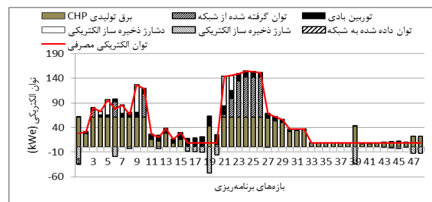
شکل (۵): سناریو ۱: تعادل توان الکتریکی در ساختمان ۱
