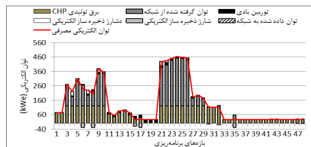
شکل (۶): سناریو ۱: تعادل توان الکتریکی در ساختمان ۲
