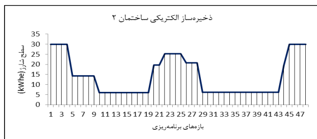
شکل (۲۲): سناریو ۳: سطح شارژ ذخیره‌ساز الکتریکی ساختمان ۲
