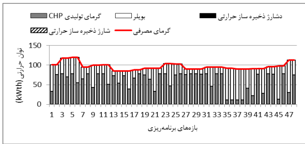
شکل (۱۳): سناریو ۳: تعادل توان حرارتی در ساختمان ۱
