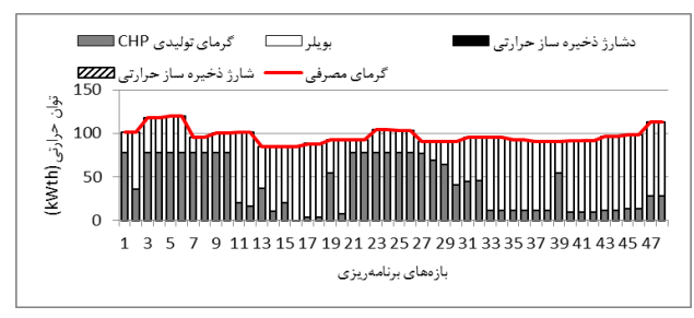
شکل (۷): سناریو ۱: تعادل توان حرارتی در ساختمان ۱
