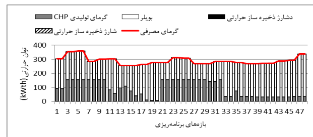
شکل (۸): سناریو ۱: تعادل توان حرارتی در ساختمان ۲
