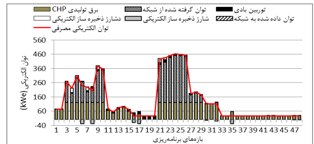
شکل (۶): سناریو ۱: تعادل توان الکتریکی در ساختمان ۲
