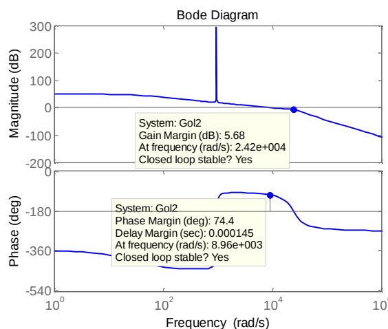
شکل (۱۲): حاشیه فاز و گین سیستم (تابع تبدیل (۲)) با گین‌های تعیین شده توسط روش پیشنهادی
