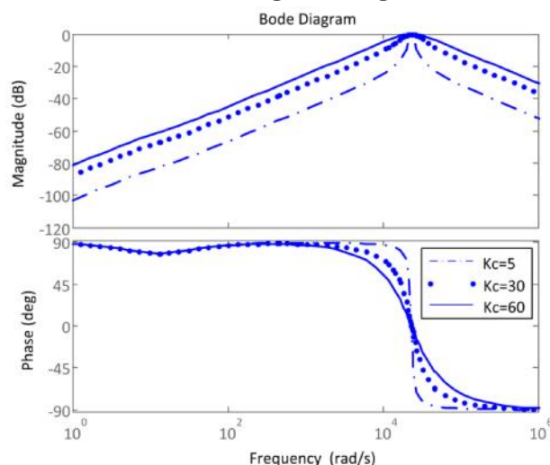
شکل (۸): تأثیر افزایش گین حلقه داخلی بر کاهش پیک رزونانس
