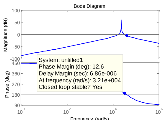
شکل (۹): دیاگرام بود حلقه داخلی با گین‌های تعیین‌شده توسط روش پیشنهادی با در نظر گرفتن یک سیکل تأخیر محاسبات
