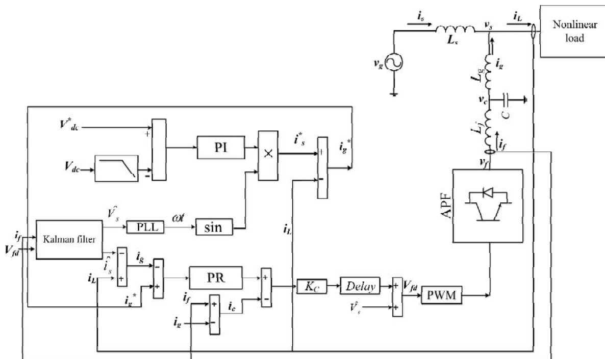
شکل (۱): دیاگرام کنترل یک فیلتر فعال با خروجی LCL با استفاده از فیلتر کالمن برای تخمین ولتاژ و جریان خط
