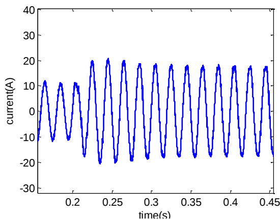
شکل (۱۴): جریان اندازه‌گیری شده خط: در لحظه‌ی t=0/2 بار از حالت خطی به غیر خطی تغییر میابد
