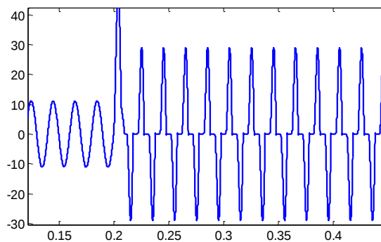
شکل (۱۶): جریان بار در t=0.2 غیر خطی می‌شود.
