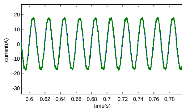
شکل (۱۷): جریان تخمین زده شده به رنگ آبی در مقایسه با جریان اندازه گیری شده به رنگ سبز در حالت دائمی
