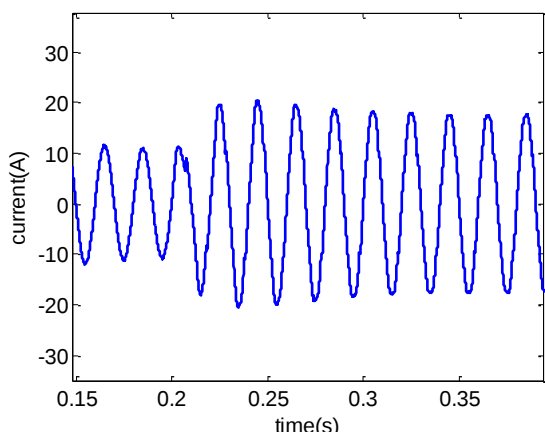
شکل (۱۵): تخمین جریان خط با تخمین زن کالمن: در لحظه‌ی t=0/2 بار از حالت خطی به غیر خطی تغییر میابد
