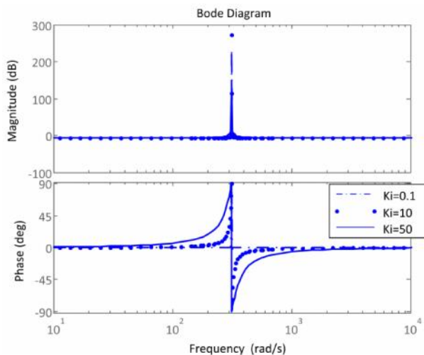
شکل (۱۱): دیاگرام بود کنترل کننده تناسبی رزونانسی با تغییر گین K_i
