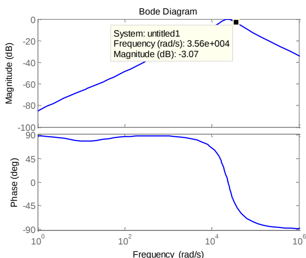
شکل (۱۰): پهنای باند حلقه بسته حلقه داخلی با گین تعیین‌شده توسط روش پیشنهادی
