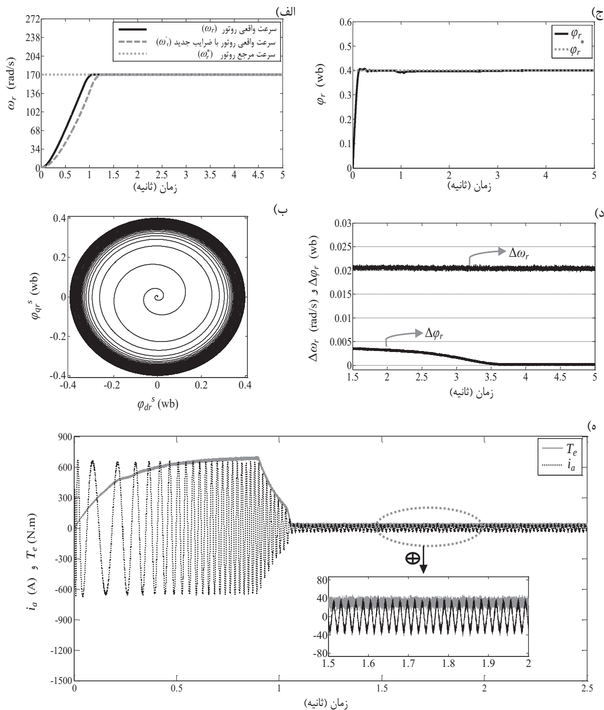
شکل (۱۶): پایداری درایو مدل پیشنهادی به ازای دو برابر شدن مقاومت استاتور در پاسخ به فرمان سرعت ۱۷۰ rad/s. الف) نمودار سرعت روتور به ازای مقادیر متفاوت K_I و K_P کنترلر عاطفی: حالت اول) همان مقادیر تعریف شده‌ی اولیه و حالت دوم) مقادیر جدید K_I=20 و K_P=30 (ب، ج) نمودار تخمین مؤلفه‌های dq شار روتور در صفحه X-Y، (د) شار روتور، (ه) نمودار خطای سرعت و شار روتور و (و) نمودار گشتاور و جریان فاز a استاتور (نمودارهای (ب)، (ج)، (د) و (ه) بر اساس همان مقادیر اولیه‌ی K_I و K_P تعریف شده، می‌باشند).
