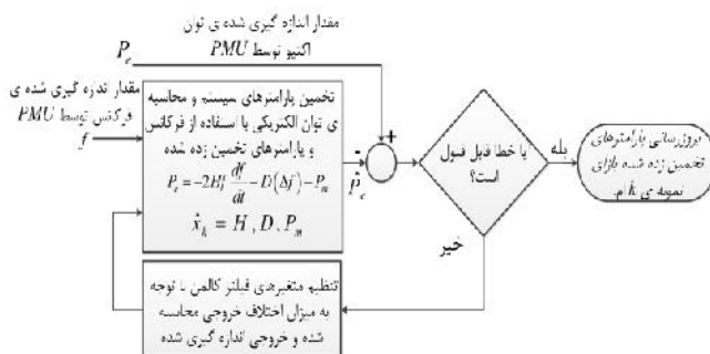
شکل (۳): الگوریتم تخمین پارامترهای الکترودمکانیکی، با استفاده از فیلتر کالمن و تکنیک بازتکرار رویداد.
