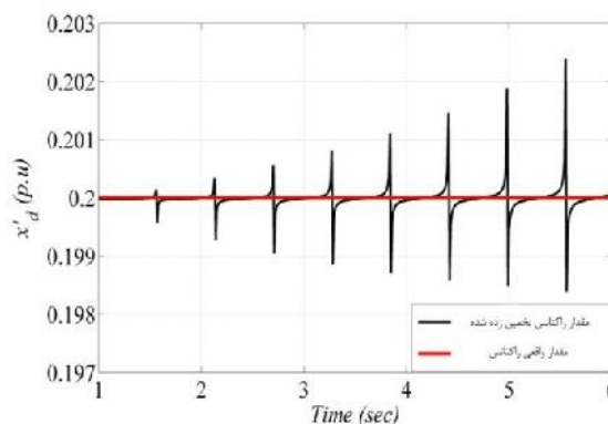
شکل (۲): مقادیر راکتانس تخمین زده شده و مقدار حقیقی آن، با استفاده از روش پیشنهادی و مشتق گیری دیفرانسیلی.
