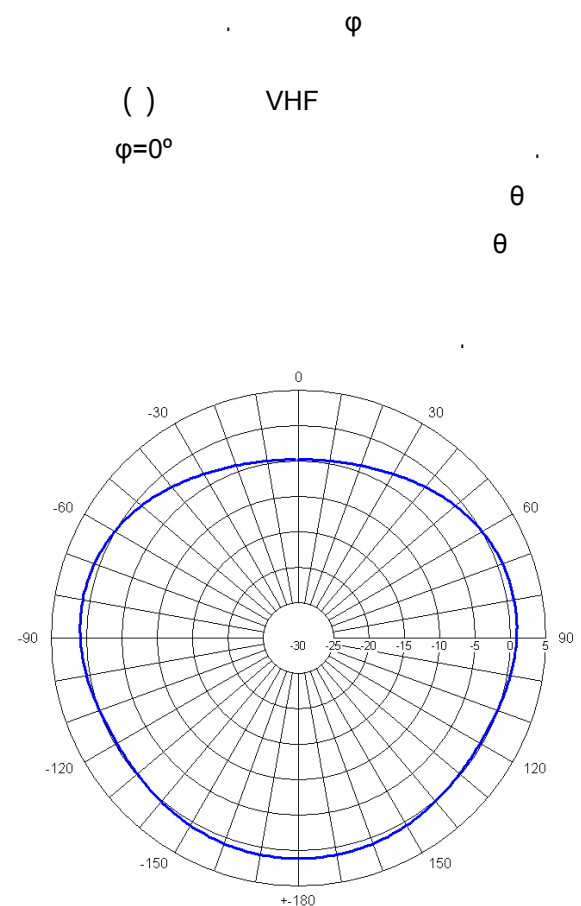
شکل (۷): گین آنتن با L=65\text{cm} و \beta=85^\circ بر حسب زاویه n در صفحه \phi=0^\circ در باند VHF
