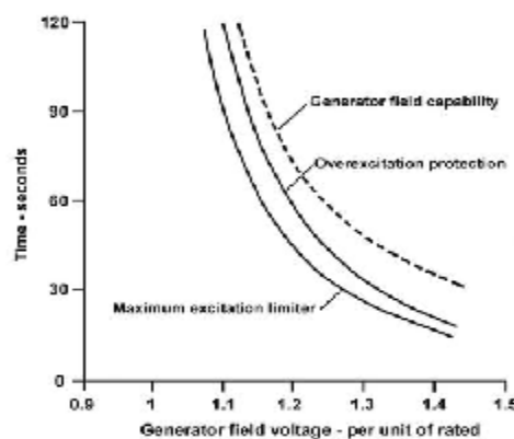
شکل ۲- منحنی اضافه بار - زمان برای تحریک ژنراتور
