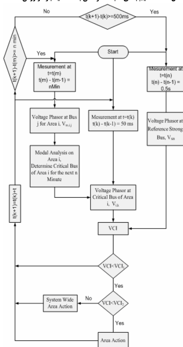
شکل ۱۷- فلوچارت الگوریتم VCI
