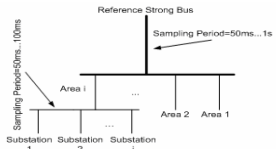
شکل ۱۱- ساختار مخابراتی پیشنهادی در روش VCI
