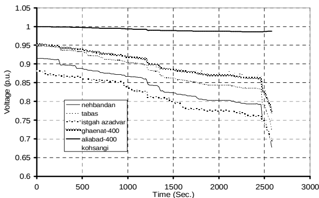
شکل ۹- ولتاژ برخی از باسهای خراسان در ناپایداری بلند مدت ولتاژ
