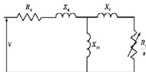
شکل ۳- مدار معادل یک موتور القایی
