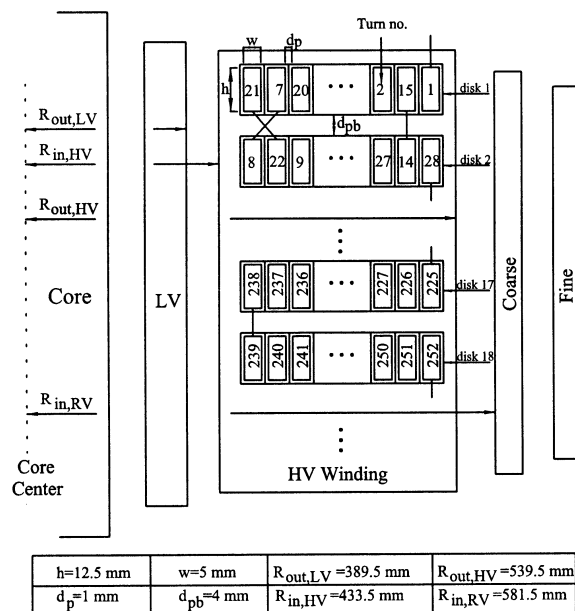
شکل (۳): ساختار ترانسفورماتور 132kV/20kV
