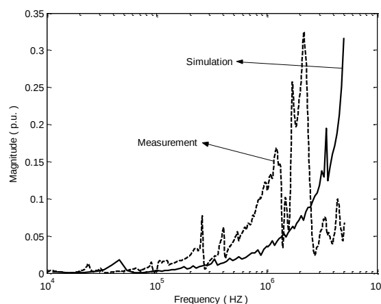
شکل (۱۱): دامنه تابع تبدیل اندازه گیری شده و محاسبه شده در حالتیکه هر دور از سیم پیچ در مدل سازی بعنوان یک خط انتقال در نظر گرفته شده باشد و ماتریس اندوکتانس با استفاده از معکوس نمودن ماتریس ظرفیت محاسبه شده باشد
