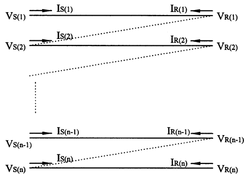
شکل (۱): مدل خط انتقال چند سیمه برای سیم پیچ
