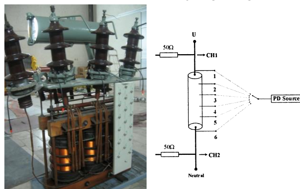
شکل (۱۳): اعمال پالسهای PD به نقاط مختلف سیم پیچ و اندازه گیری آنها در دو انتهای سیم پیچ
