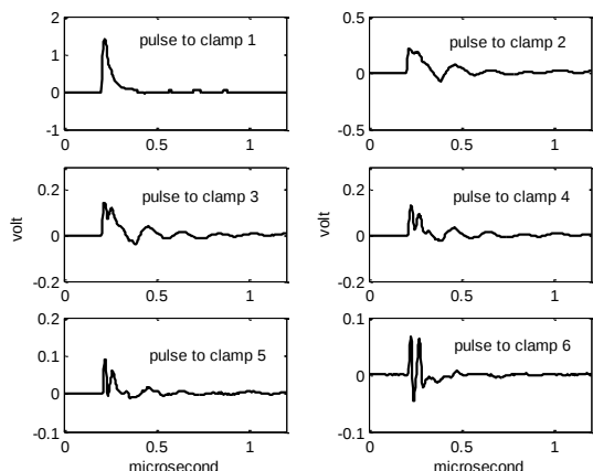
شکل (۱۴): پالسهای اندازه گیری شده در ابتدای سیم پیچ
