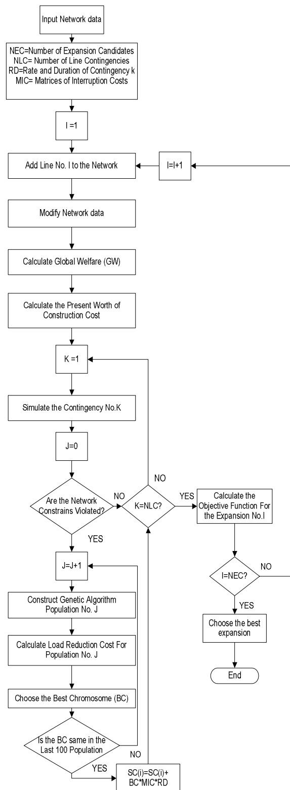
شکل (1): فلوچارت بدست آوردن تابع هدف برای سناریو های مختلف توسعه
