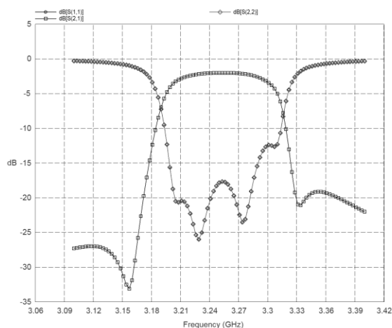
شکل (۶): پاسخ فرکانسی حاصل از شبیه‌سازی فیلتر از جنس مس روی زیر لایه از جنس \text{LaAlO}_3 به ضخامت 1mm
