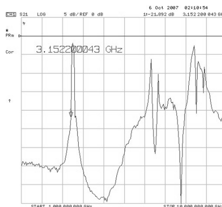
شکل (۱۱): پاسخ فرکانسی پهن باند فیلتر (span=9GHz)
