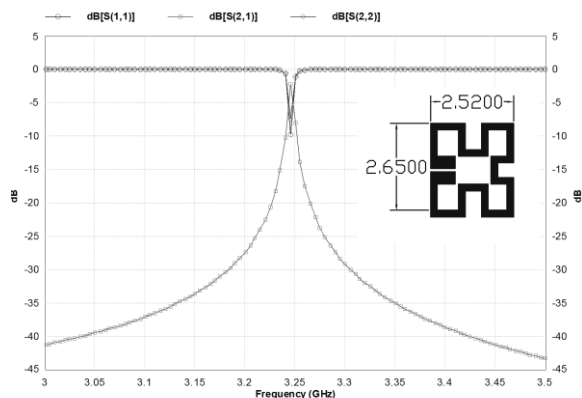
شکل (۱): شمای مشدد فشرده طراحی شده و پاسخ فرکانسی آن
