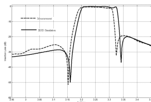
شکل (۱۲): مقایسه پاسخ فرکانسی اندازه‌گیری شده و حاصل از شبیه
