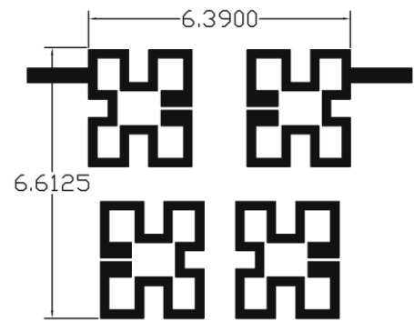
شکل (۴): طرح فیلتر مایکرواستریپ میانگذر ۴ قطبی
