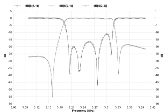
شکل (۵): پاسخ فرکانسی حاصل از شبیه‌سازی فیلتر میانگذر
